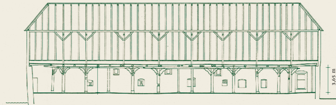
Seitenansichten „Roggenhaus“
